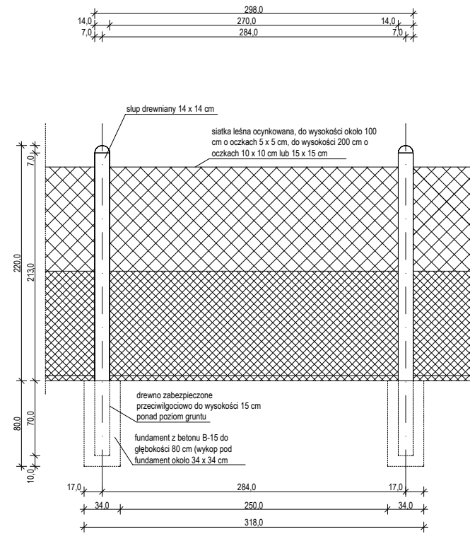
Ogrodzenie typ E - przesło podstawowe
