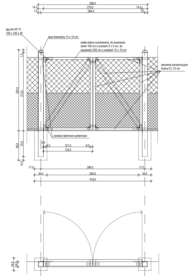
Ogrodzenie typ F - brama dwuskrzydłowa
